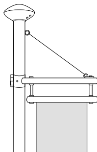
BMAL - Banier op alu mast
