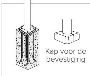
FSB - bevestiging in de grond met kantelvoet
