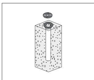
FSF - bevestiging in de grond met grondkoker
