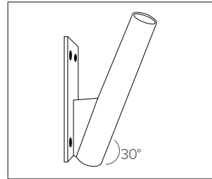
B48S - enkele muurkoker, schuin
